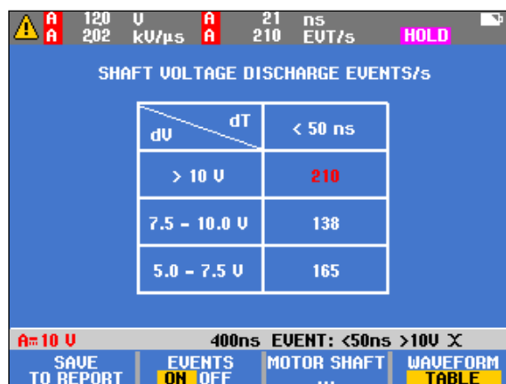
Recuentos de eventos de descarga de tensión del eje del motor
